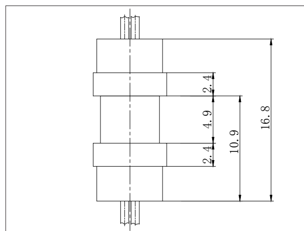
左视图
