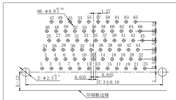
J30J-66ZKW
