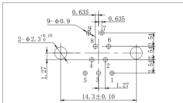
J30J-9TJN、TJN4、TJN8
