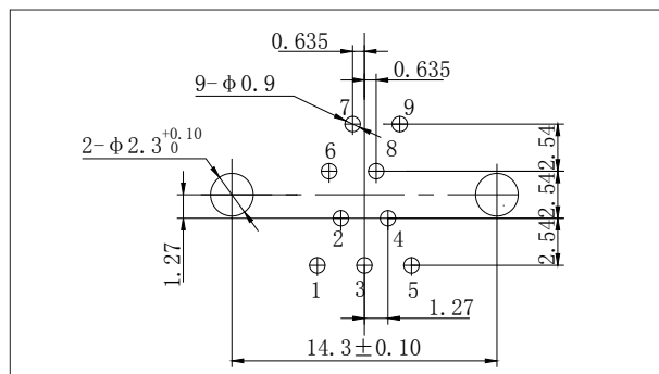
J30J-9ZKN、ZKN3、ZKN4
