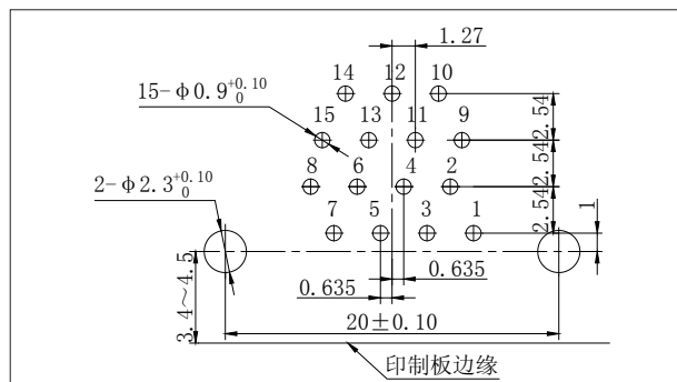
J30J-15TJW-Q8
