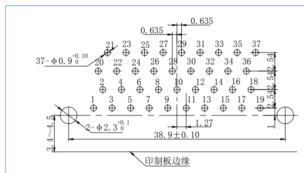
J30JC-37ZKW-Q
