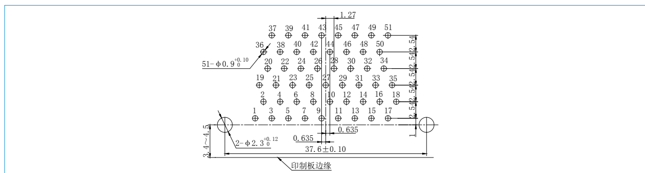
J30JC-51ZKW-Q
