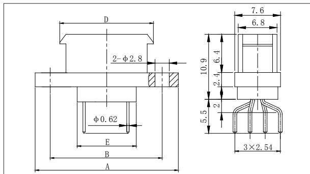
J30JA-9 ~ 37 ZKN
