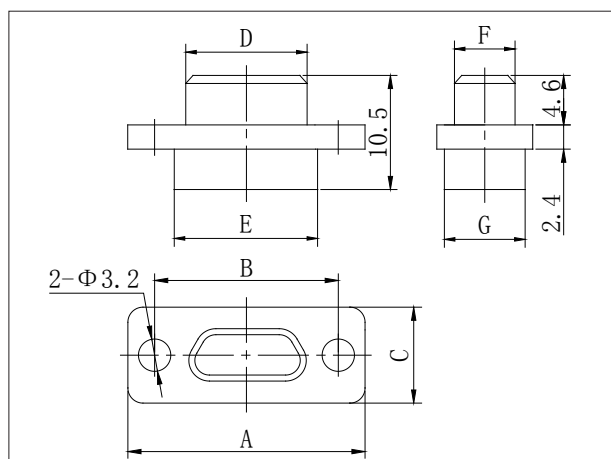
J30J- □ TJ-Q
