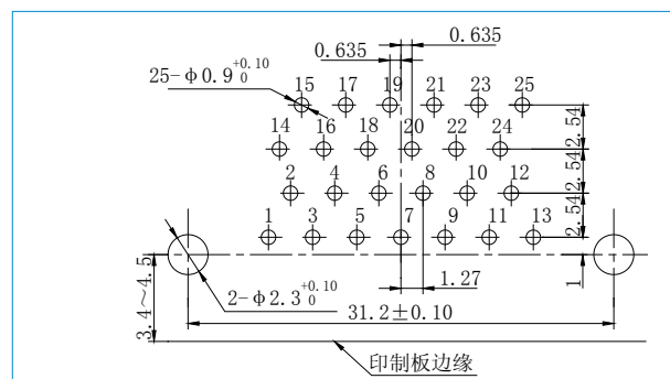
J30JC-25ZKW-Q
