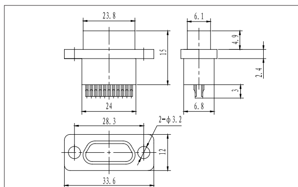
J30JM-31ZKS
