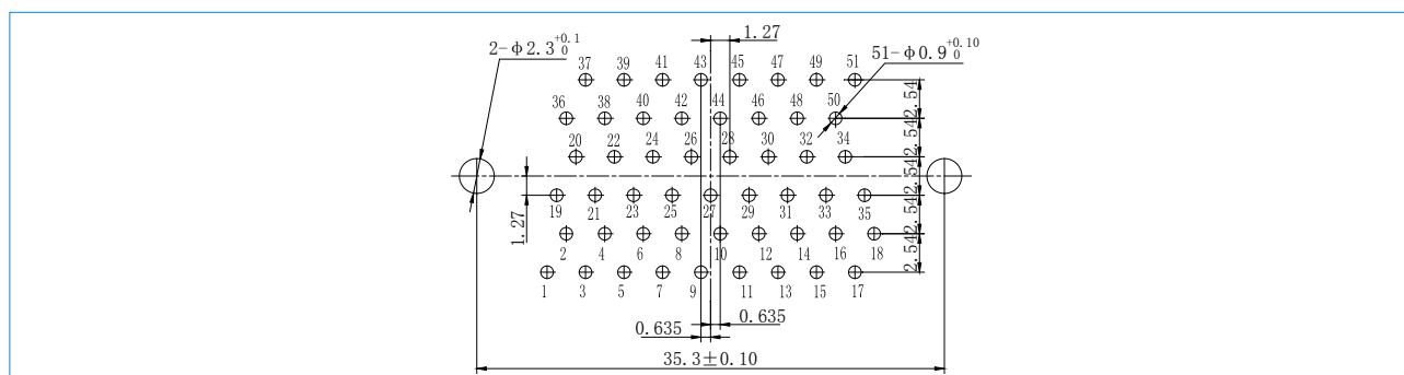
J30JA-51ZKN
