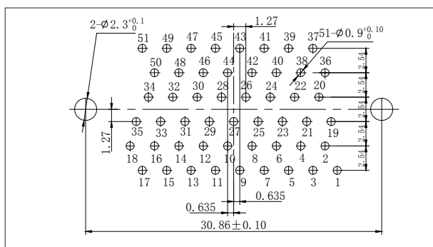
J30J-51TJN、TJN4
