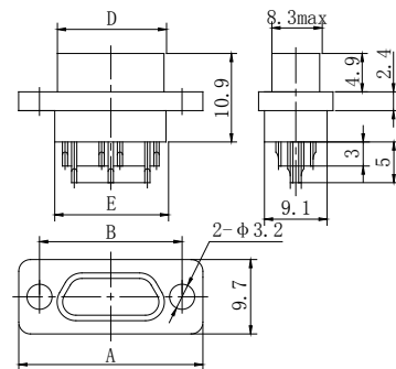
J30J-74, 100ZKS
