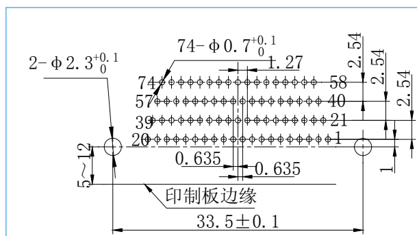
J30J-74TJW-J
