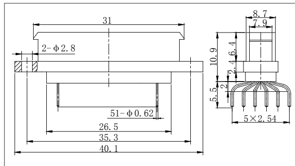
J30JA-51ZKN
