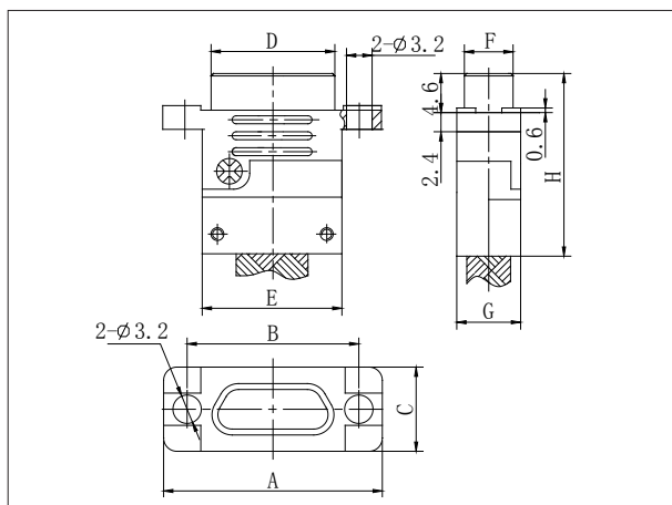
J30J- □ TJ-AD
