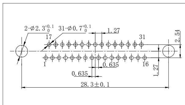
J30J-31ZKN-J、ZKN4-J
