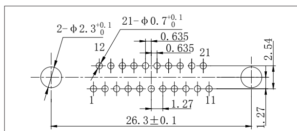
J30JA-21ZKN-J
