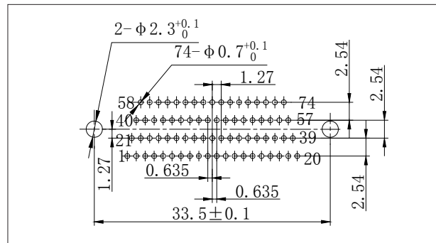
J30J-74ZKN-J、ZKN4-J
