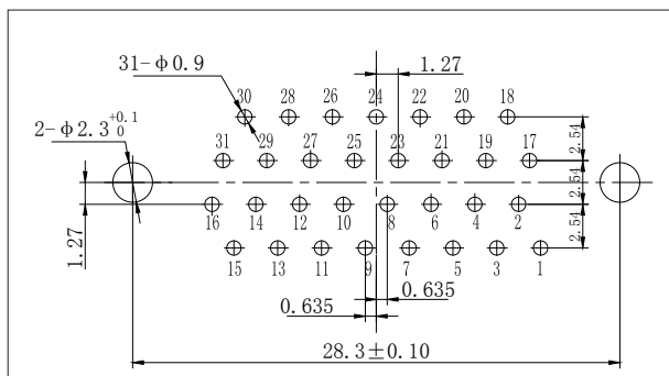
J30J-31TJN、TJN4、TJN8
