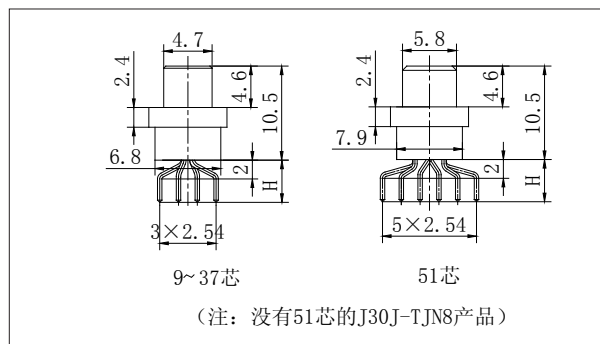
各芯数插头合件的左视图
