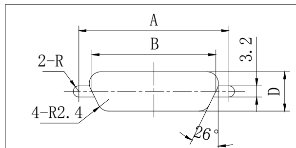
板后安装开孔尺寸
