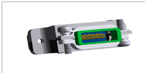
从线夹尾端看到的立体图
