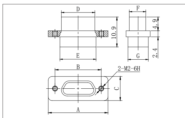
J30JD-XZK
