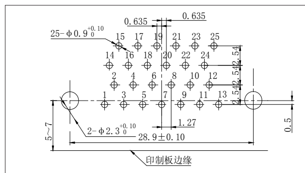
J30JA-25ZKW
