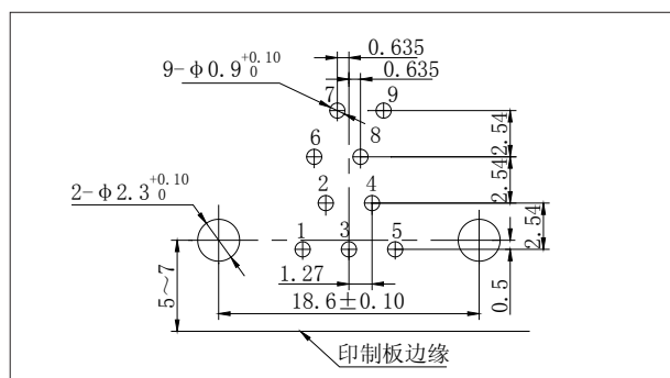
J30JA-9ZKW
