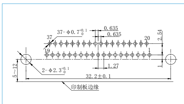
J30J-37TJW-J
