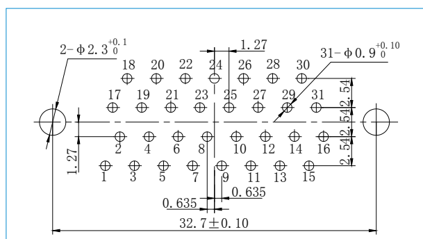
J30JA-31ZKN
