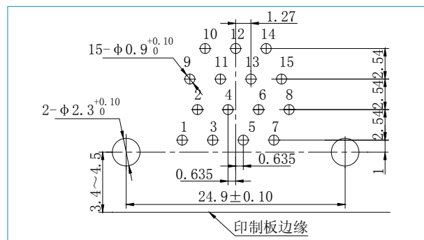
J30JC-15ZKW-Q
