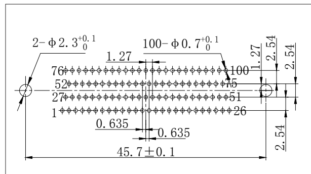
J30J-100ZKN-J、ZKN4-J
