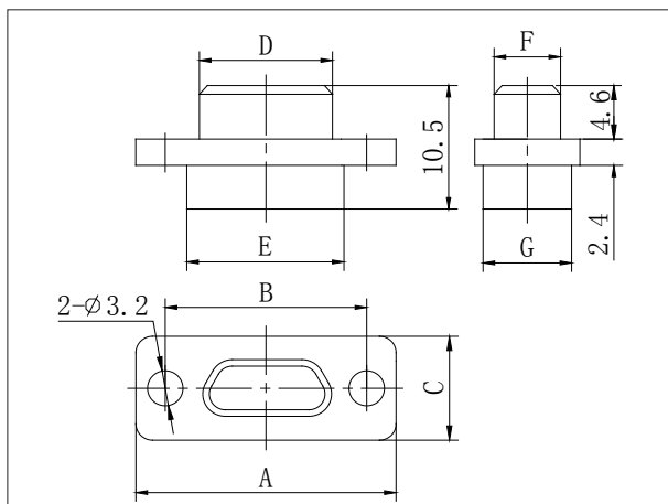
J30J- □ TJ
