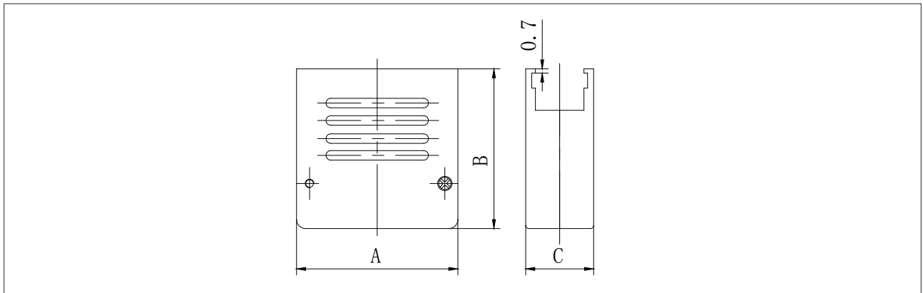
J30J-xA2 线夹合件
