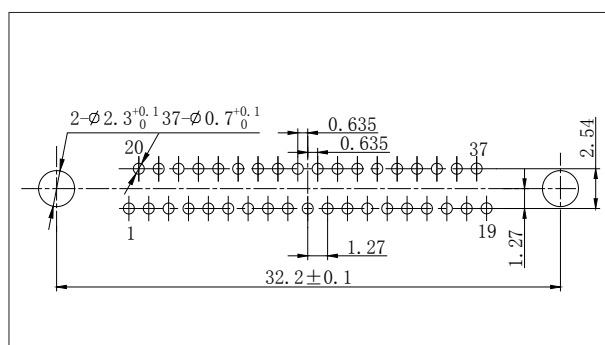
J30J-37ZKN-J、ZKN4-J
