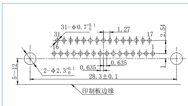
J30J-31TJW-J
