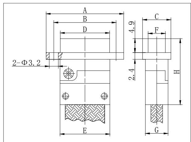
J30J-9~100ZK-AQ8
