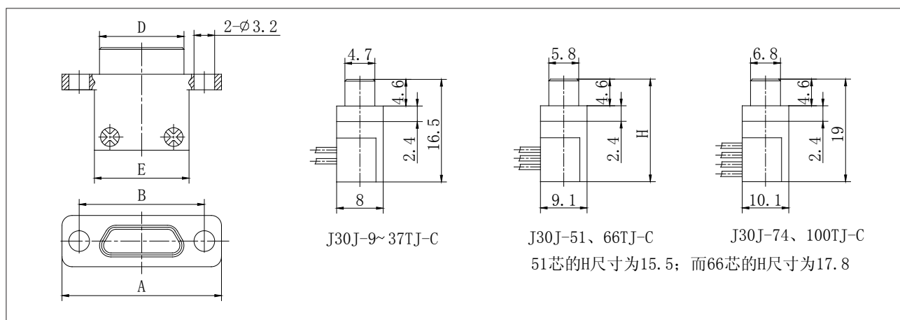
各芯数插座合件左视图
