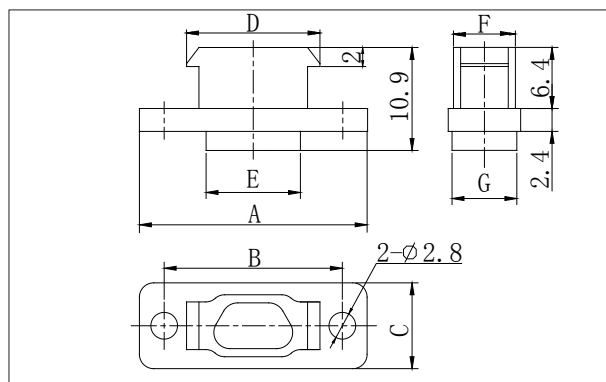
J30JA-XZK
