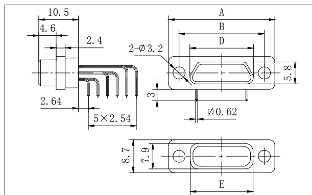
J30J-51、66TJW
