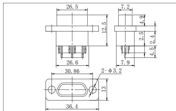
J30JM1-51ZKS
