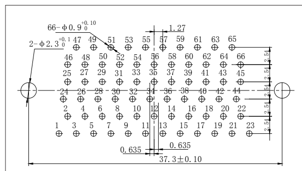
J30J-66ZKN、ZKN3、ZKN4
