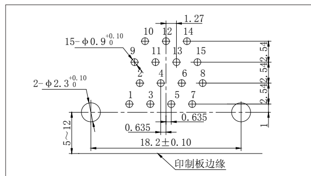
J30J-15ZKW
