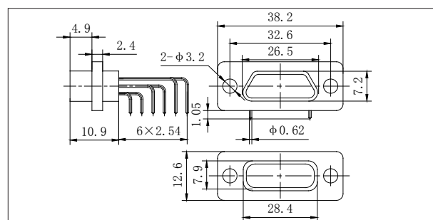
J30J-51ZKW-Q8
