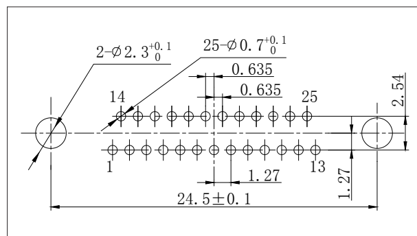
J30J-25ZKN-J、ZKN4-J
