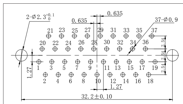
J30J-37ZKN、ZKN3、ZKN4
