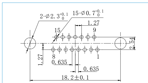
J30J-15TJN-J
