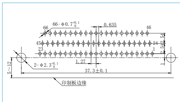
J30J-66TJW-J
