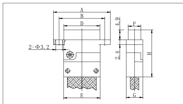
J30J- □ ZK-A
