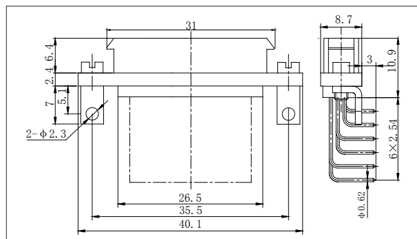
J30JA-51ZKW
