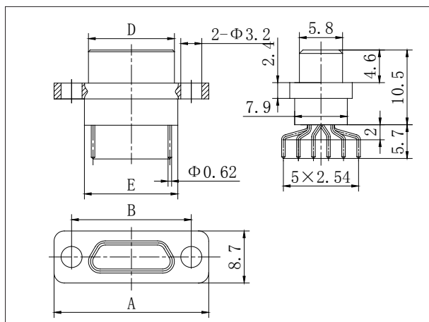
J30J-51、66TJN
