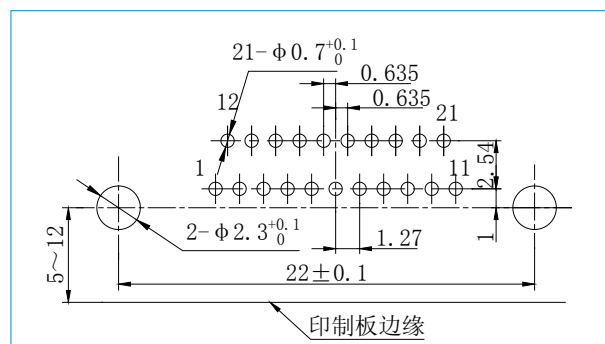
J30J-21ZKW-J
