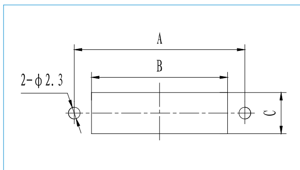
板前安装开孔尺寸
