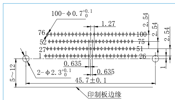
J30J-100ZKW-J
