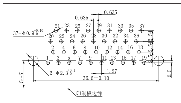
J30JA-37ZKW
