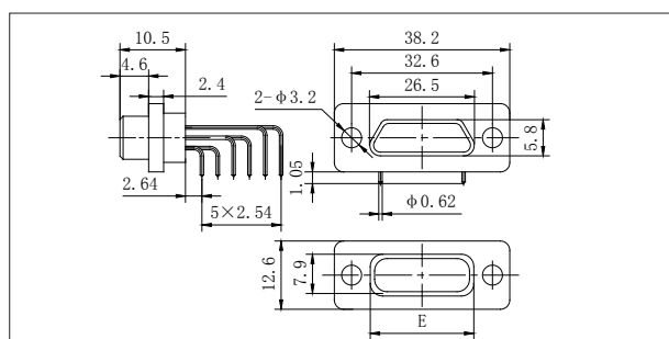
J30J-51TJW-Q8
