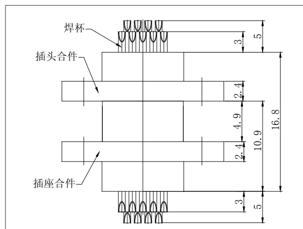
J30J-51~100 芯
