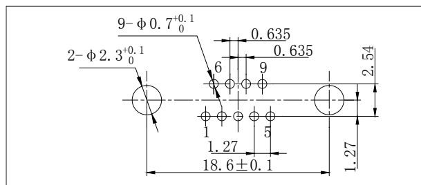
J30JA-9ZKN-J
