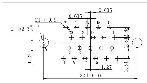
J30J-21TJN、TJN4、TJN8
