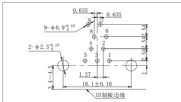
J30J-9TJW-Q8
