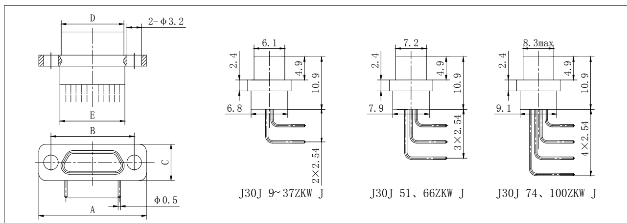
各芯数插头合件的左视图
