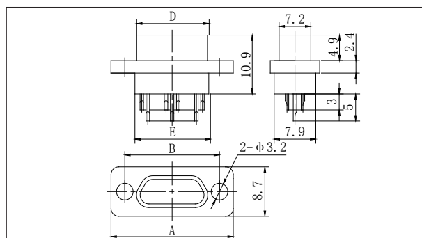
J30J-51, 66ZKS
