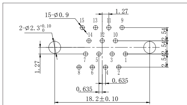
J30J-15TJN、TJN4、TJN8
