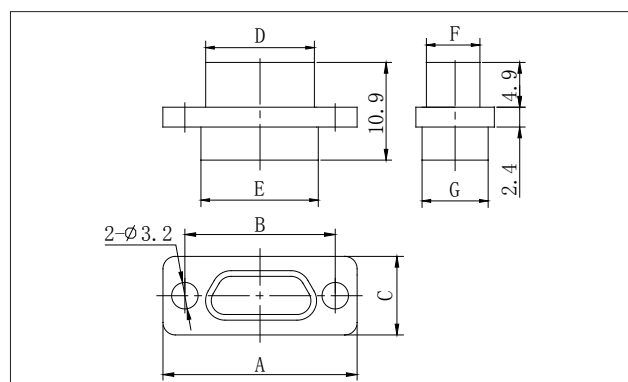
J30J- □ ZK-Q8
