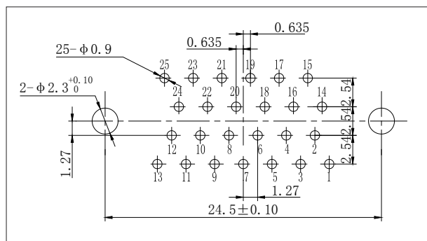
J30J-25TJN、TJN4、TJN8
