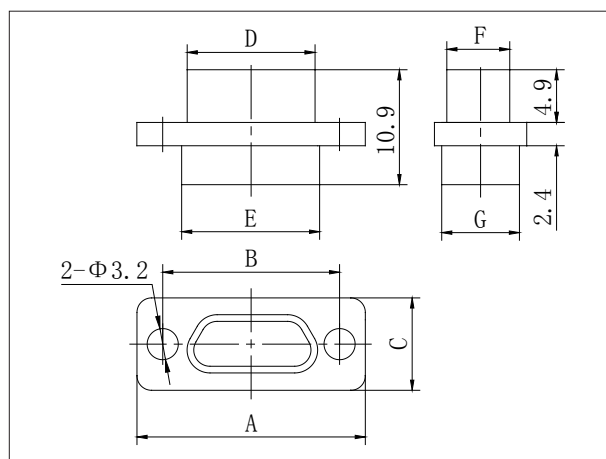
J30J- □ ZK-Q
