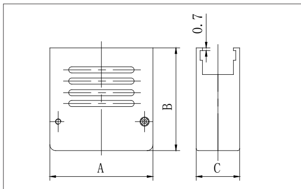
J30J-× A1 线夹合件
