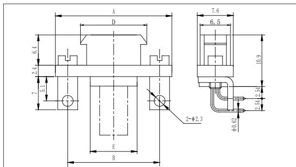
J30JA-9 ~ 37ZKW-J
