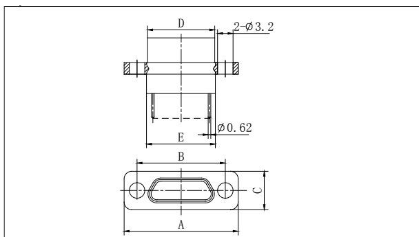
J30J-9~51ZKN3/J30J-9~51ZKN4
