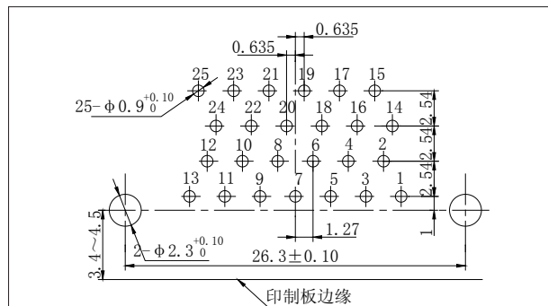
J30J-25TJW-Q8
