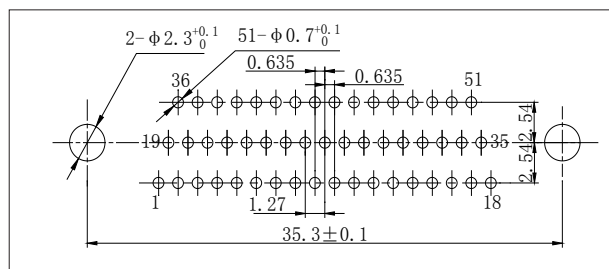
J30JA-51ZKN-J
