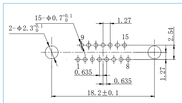
J30J-15ZKN-J、ZKN4-J
