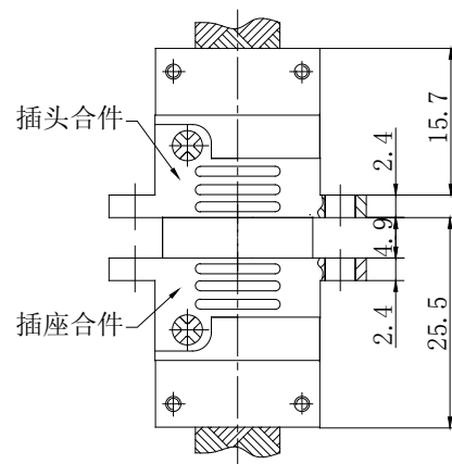
J30J-74~100 芯
