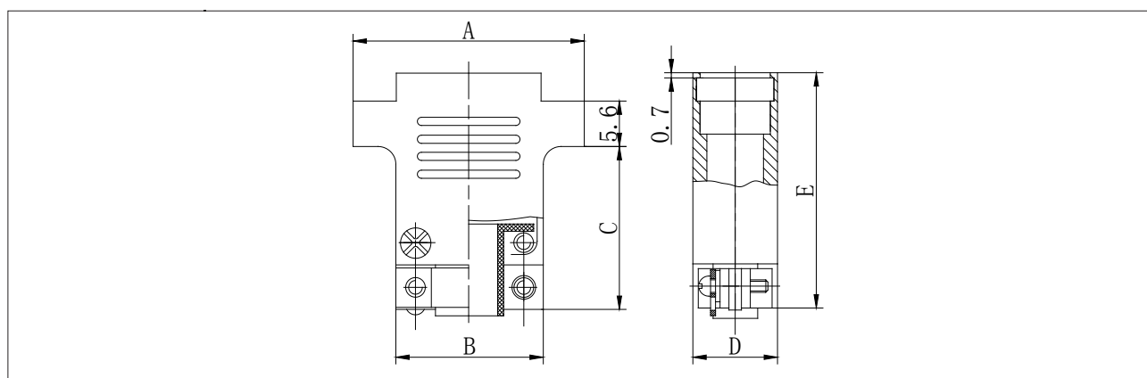
A3 型线夹合件的尺寸
