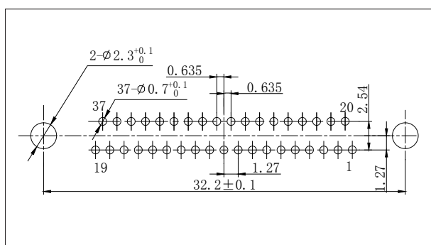
J30J-37TJN-J
