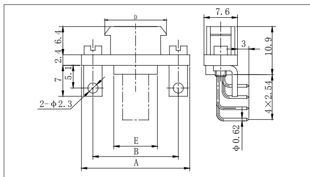
J30JA-9 ~ 37ZKW
