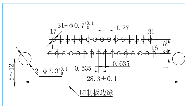
J30J-31ZKW-J
