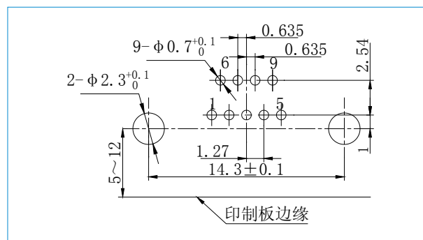
J30J-9ZKW-J
