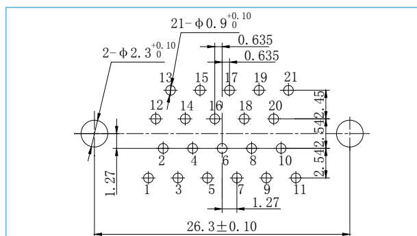
J30JA-21ZKN
