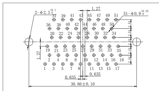
J30J-51ZKN、ZKN3、ZKN4
