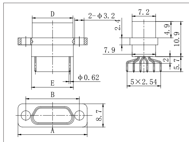
J30J-51、66ZKN
