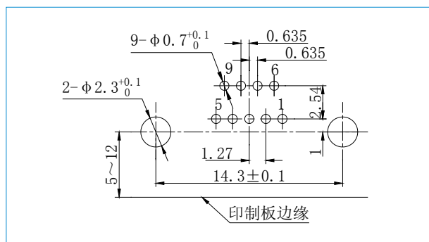
J30J-9TJW-J
