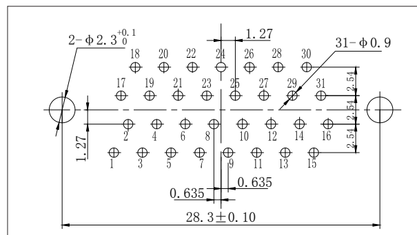
J30J-31ZKN、ZKN3、ZKN4
