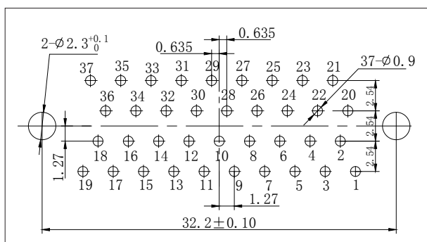
J30J-37TJN、TJN4、TJN8
