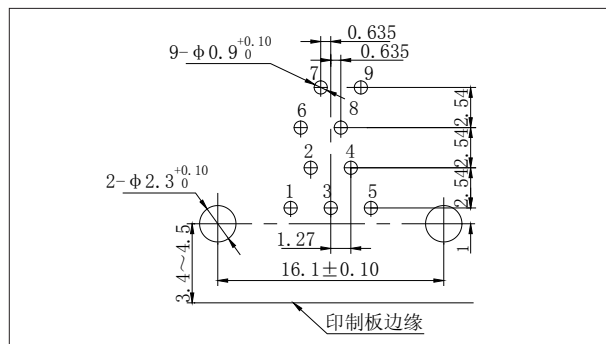
J30J-9ZKW-Q8
