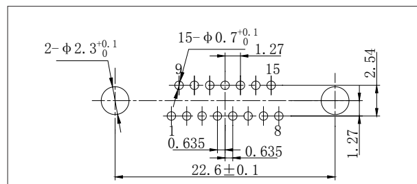
J30JA-15ZKN-J
