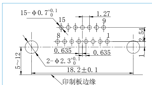
J30J-15TJW-J
