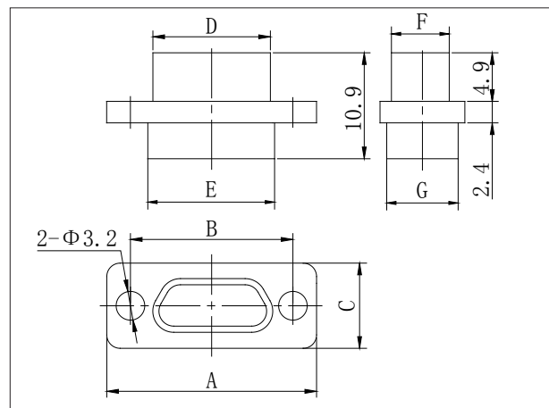
J30J- □ ZK
