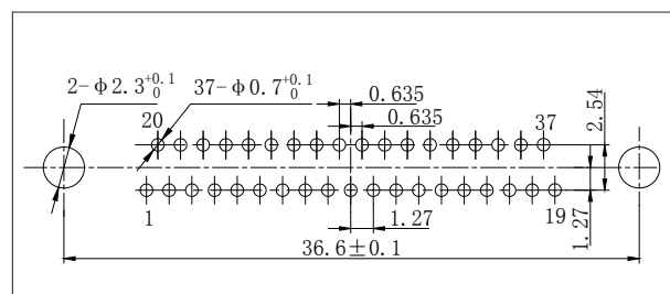
J30JA-37ZKN-J
