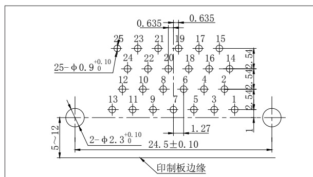
J30J-25TJW
