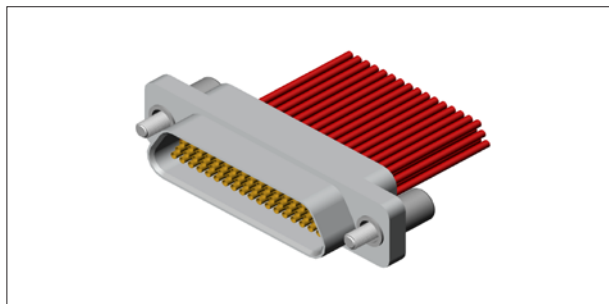
组装示意图
