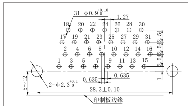
J30J-31ZKW
