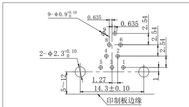
J30J-9TJW
