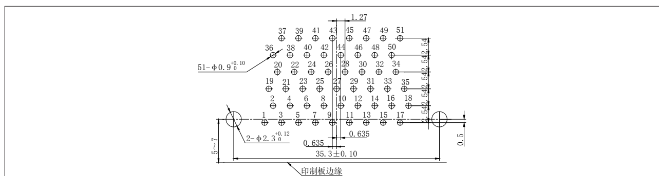
J30JA-51ZKW
