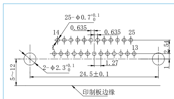
J30J-25ZKW-J
