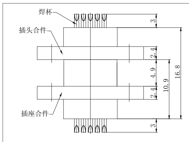
J30J-9~37 芯
