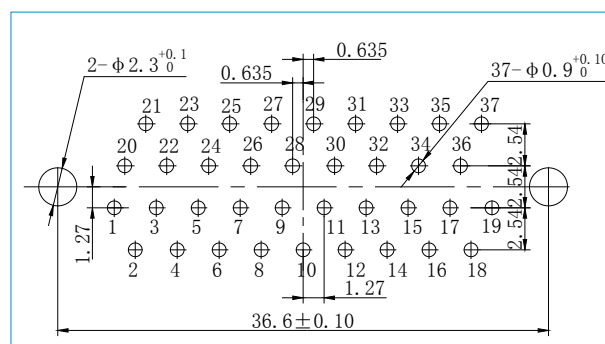
J30JA-37ZKN
