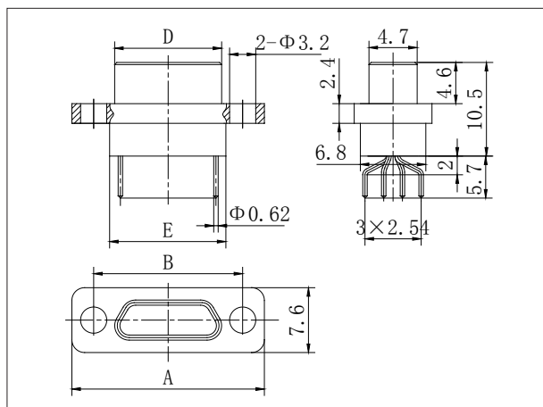
J30J-9~37TJN
