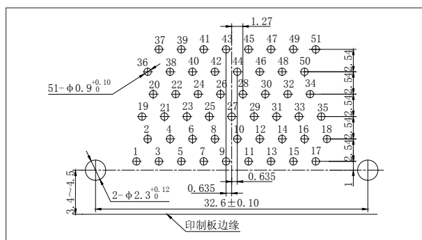
J30J-51ZKW-Q8
