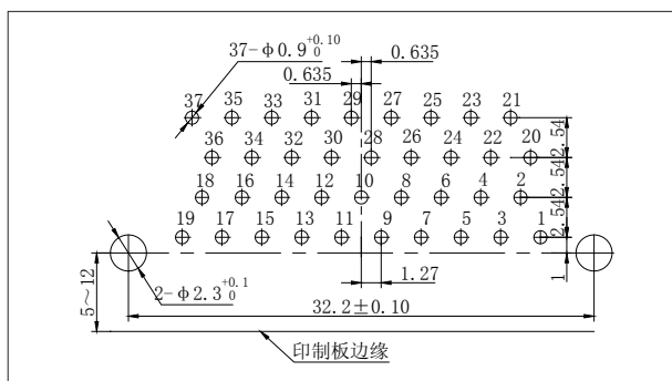
J30J-37TJW
