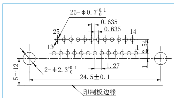
J30J-25TJW-J
