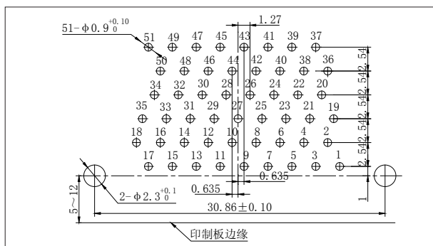
J30J-51TJW
