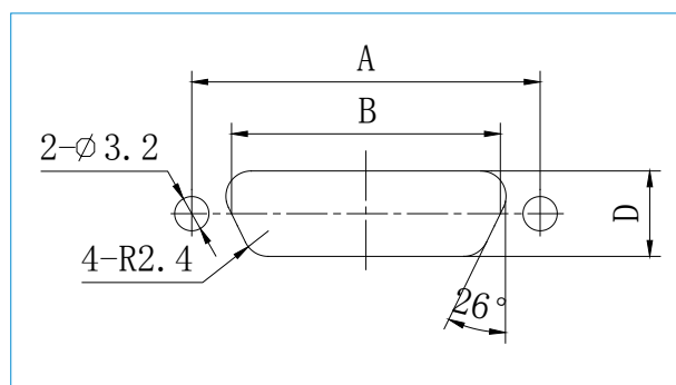
板后安装开孔尺寸
