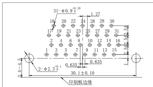
J30J-31ZKW-Q8
