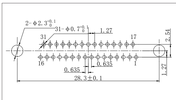
J30J-31TJN-J
