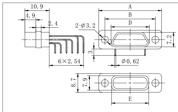
J30J-51、66ZKW
