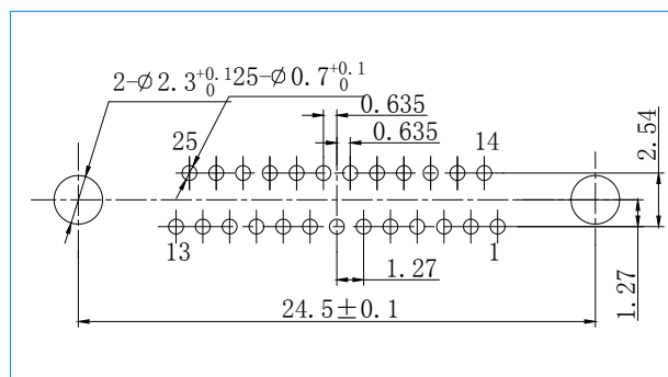
J30J-25TJN-J
