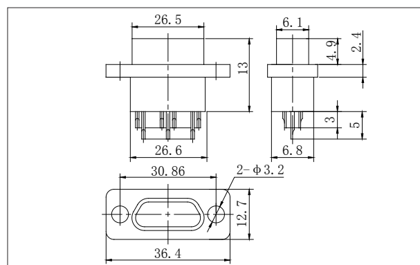
J30JM-51ZKS
