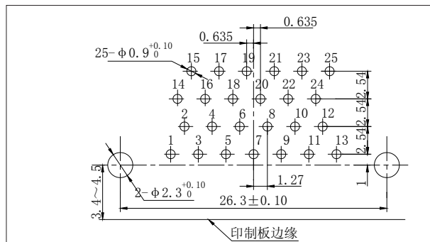
J30J-25ZKW-Q8
