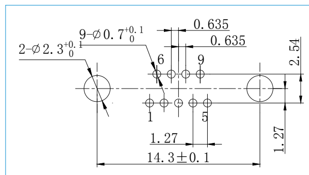
J30J-9ZKN-J、ZKN4-J
