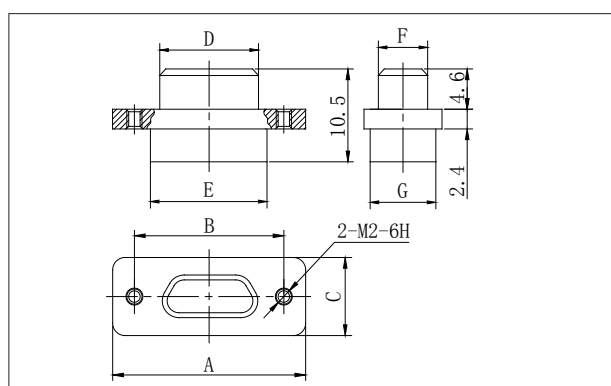
J30JD-XTJ
