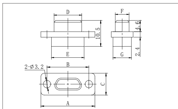
J30J- □ TJ-Q8
