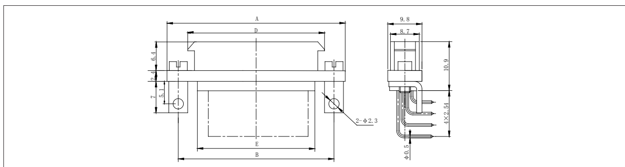
J30JA-74、100ZKW-J
