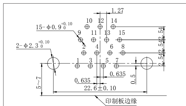
J30JA-15ZKW
