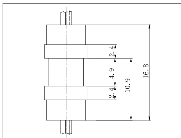
左视图
