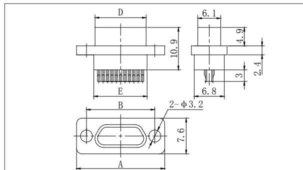
J30J-9~37ZKS
