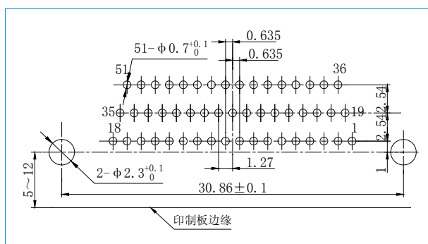
J30J-51TJW-J
