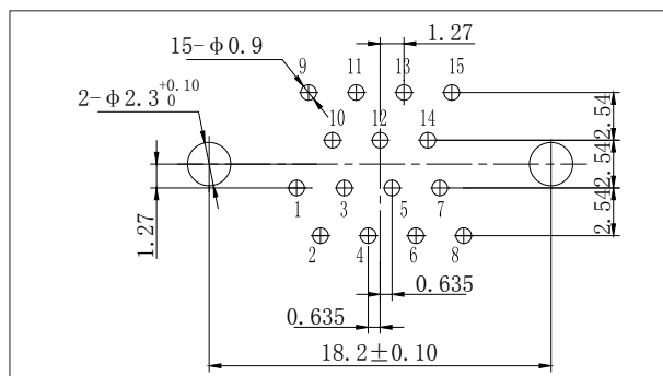
J30J-15ZKN、ZKN3、ZKN4
