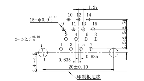
J30J-15ZKW-Q8
