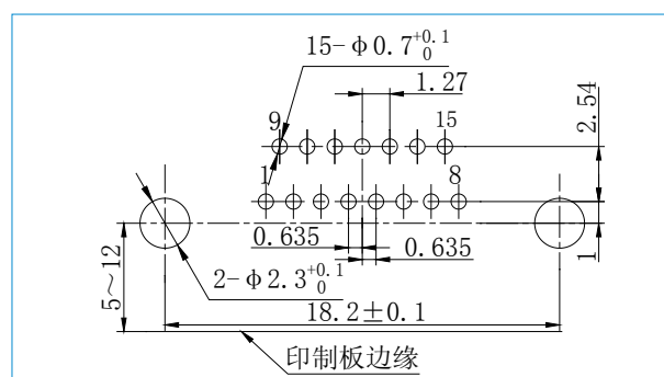
J30J-15ZKW-J
