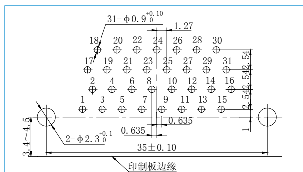
J30JC-31ZKW-Q
