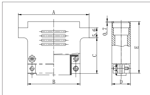
J30J-× A3 线夹合件
