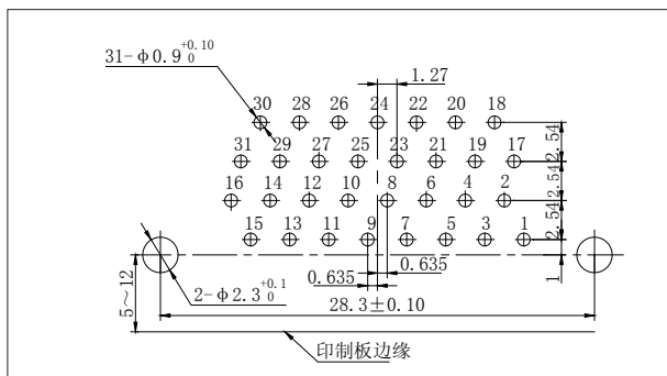
J30J-31TJW
