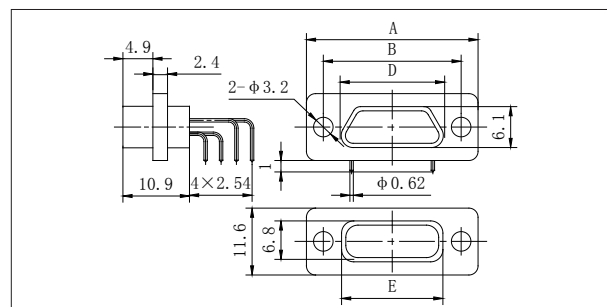
J30J-9~37ZKW-Q8
