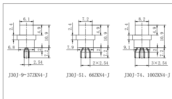
各芯数插座合件左视图
