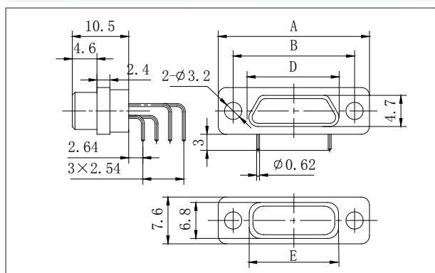
J30J-9~37TJW
