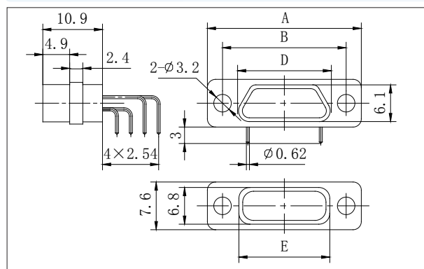
J30J-9~37ZKW
