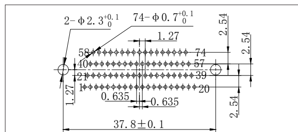
J30JA-74ZKN-J
