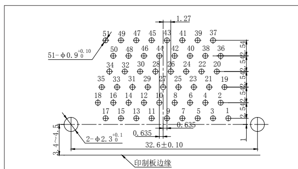
J30J-51TJW-Q8
