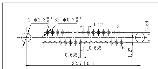
J30JA-31ZKN-J
