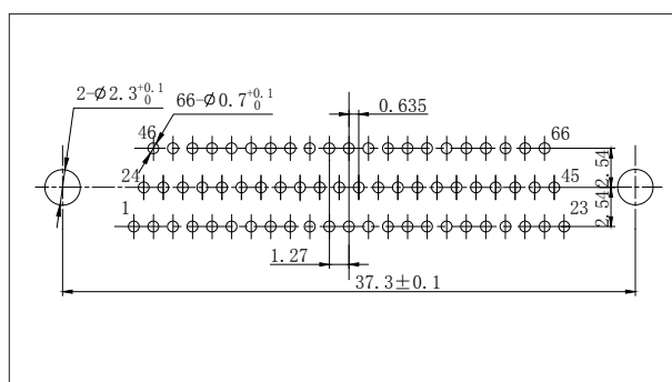
J30J-66ZKN-J、ZKN4-J
