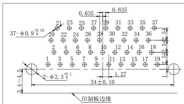
J30J-37ZKW-Q8
