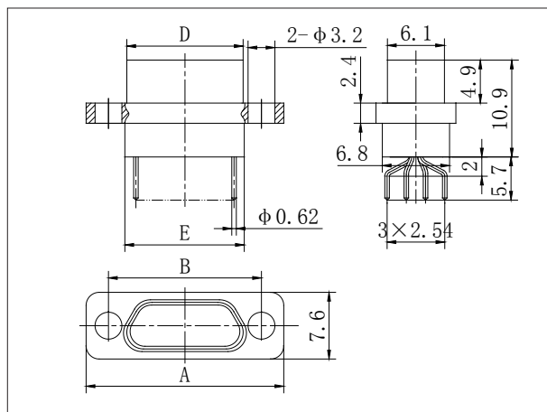
J30J-9~37ZKN
