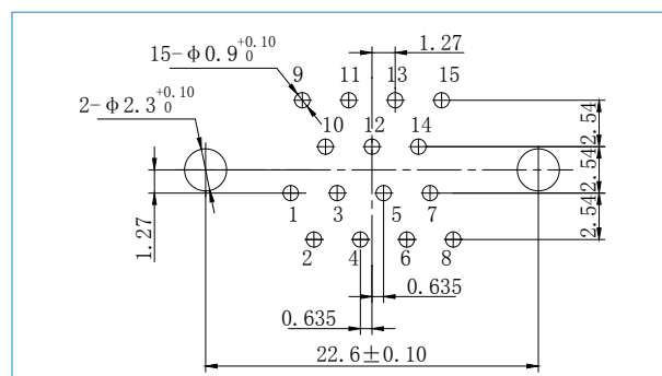
J30JA-15ZKN
