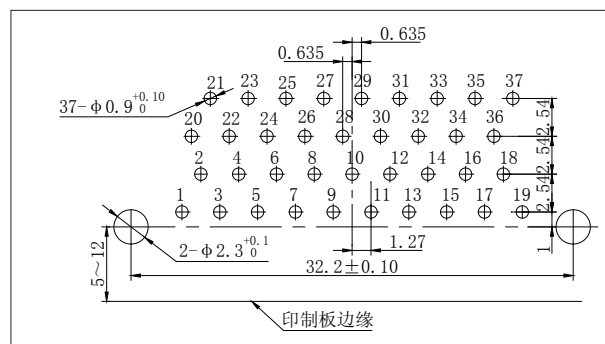
J30J-37ZKW
