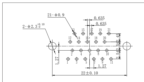
J30J-21ZKN、ZKN3、ZKN4
