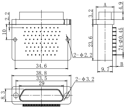
产品外形尺寸图
