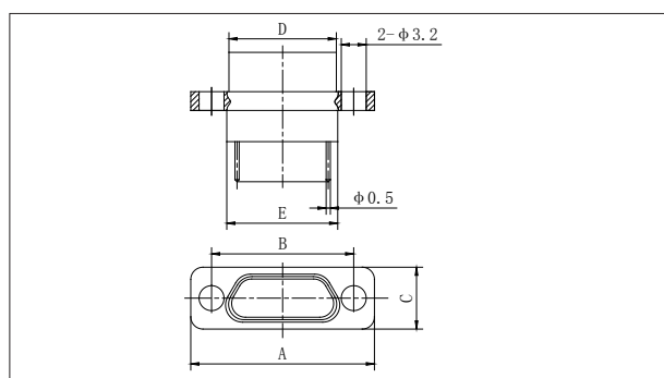
J30J-9~100ZKN4-J
