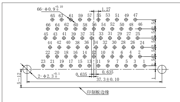
J30J-66TJW
