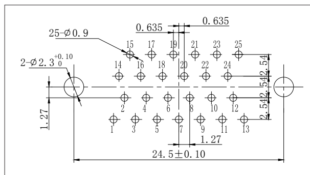
J30J-25ZKN、ZKN3、ZKN4
