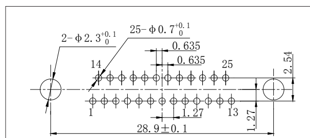
J30JA-25ZKN-J
