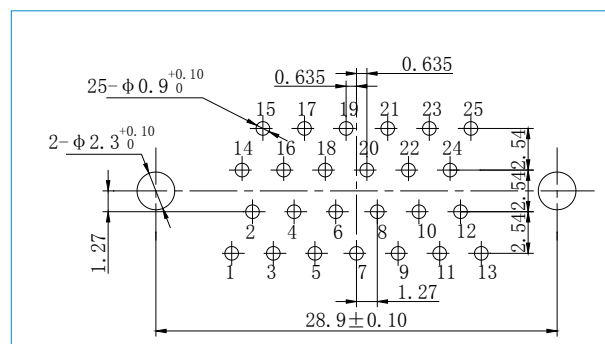
J30JA-25ZKN
