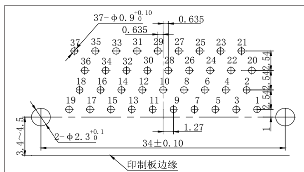
J30J-37TJW-Q8
