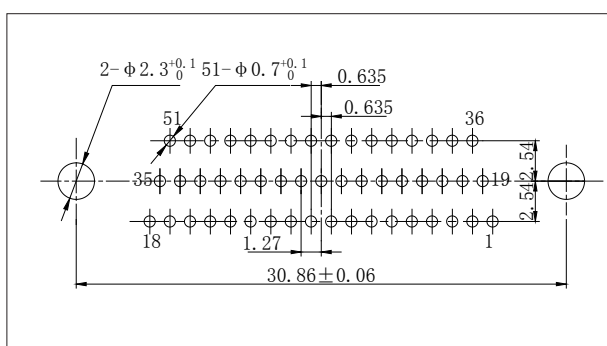
J30J-51TJN-J
