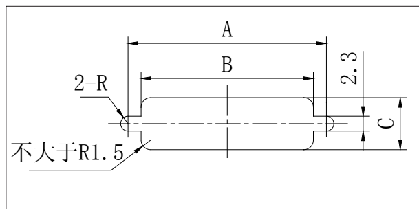
板前安装开孔尺寸
