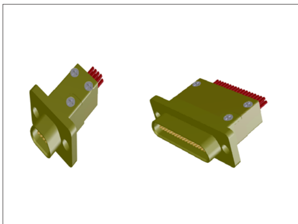
J30J-9ZK-GA (11.6)
