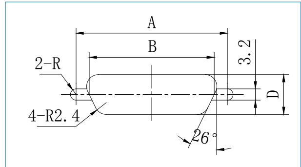
板后安装开孔尺寸
