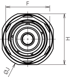
8D7 Jam nut receptacle
